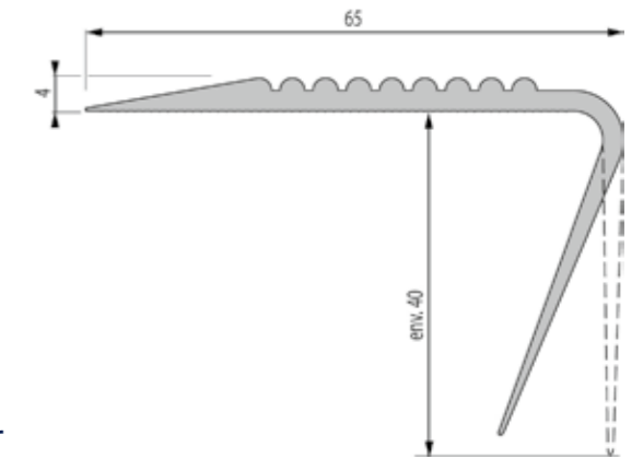
Nez de marche PVC pose rapportée à coller
